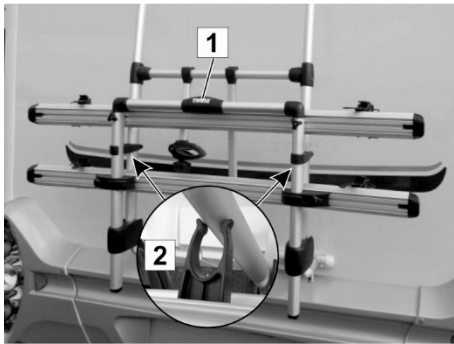
Fig. 22 : Déplier le porte-vélos
