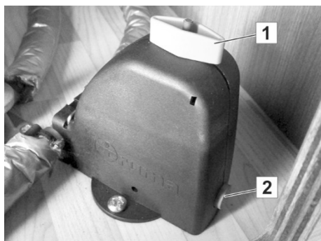
Fig. 156 : Vanne de vidange de sécurité ouverte
