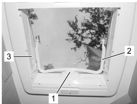
Fig. 113 : Manœuvre du Midi Heki / Mini Heki plus
