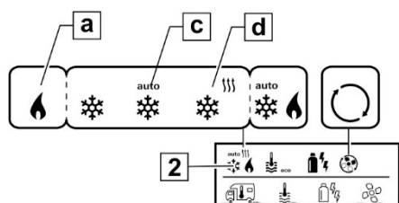
Fig. 124 : Symbole de la température ambiante
