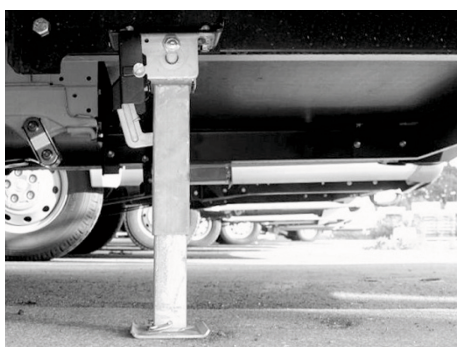
Fig. 14: Vérin arrière, en place
