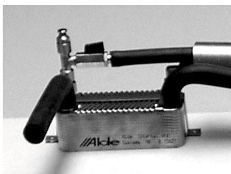
Fig. 87 : Echangeur de chaleur ALDE
