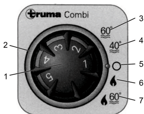
Fig. 118 : Unité de commande TRUMA pour chauffage et production d'eau chaude
