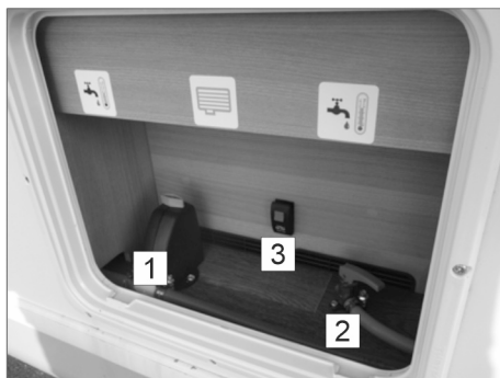
Fig. 92 : Vannes de vidange
