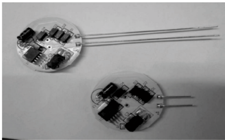
Fig. 196 : Raccourcir les contacts
