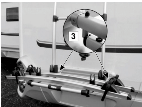
Fig. 23 : Enclencher les arrêtoirs
