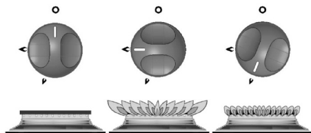
Fig. 186 : Positions des boutons : ARRÊT, grande flamme, petite flamme
