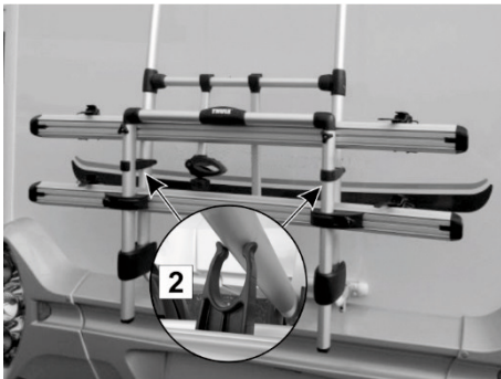
Fig. 26 : Ramener le porte-vélos vers le haut
